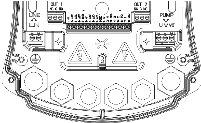
Resim 1: Elektrik Bağlantıları
