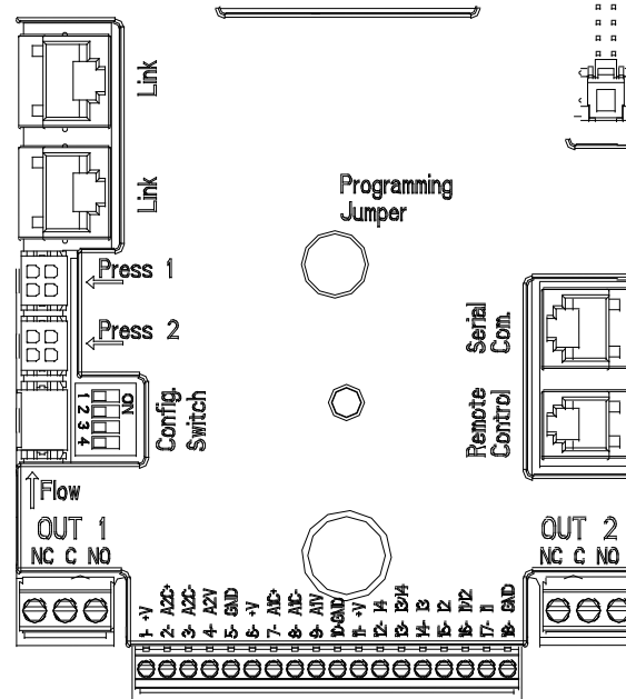
Slika 3: Priključki
