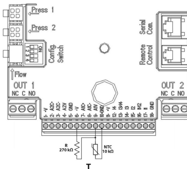
Figura 8: Collegamento sensore NTC per misura temperatura T
