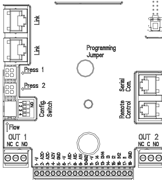
Figura 3: Connessioni
