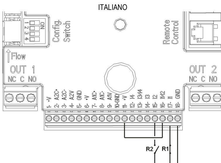
Figura 4: Esempio Collegamento Ingressi Digitali Start/Stop ed Economy
