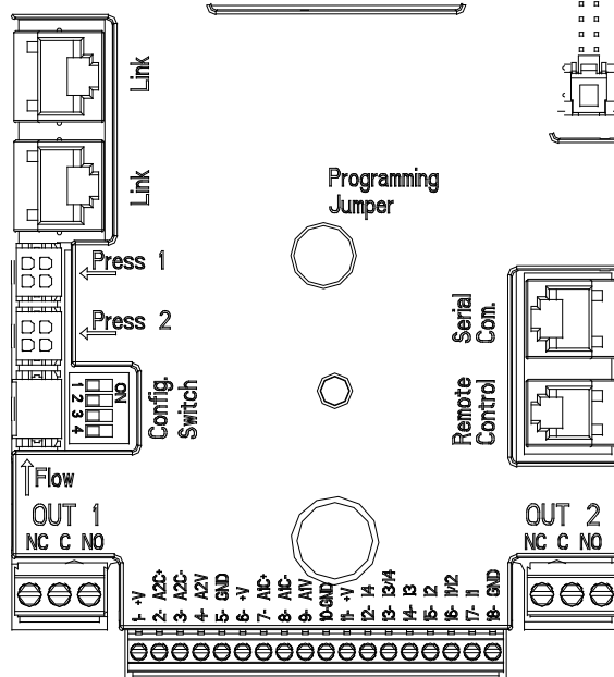
Фиг. 3: Свързвания
