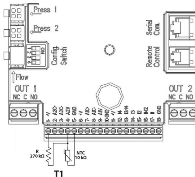
Figura 7: Conexiune senzor NTC pentru măsurarea temperaturii T1
