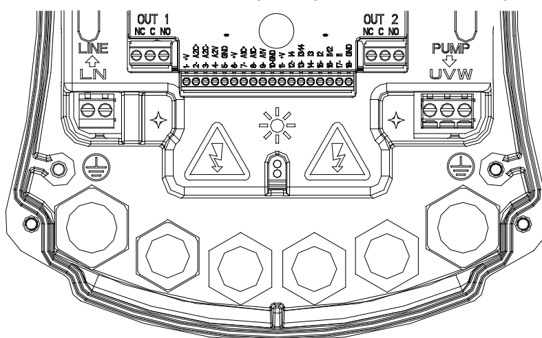
Fig. 1: Elanslutning
