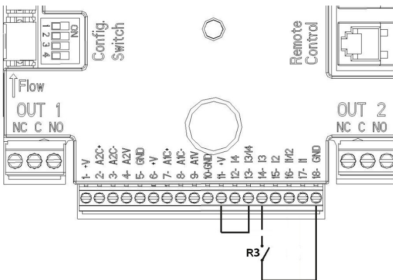
Afbeelding 5: Aansluitvoorbeeld digitale ingang Quick Start
