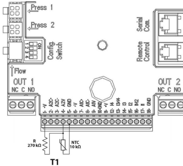
Resim 7: T1 sıcaklık ölçümü için NTC sensör bağlantısı
