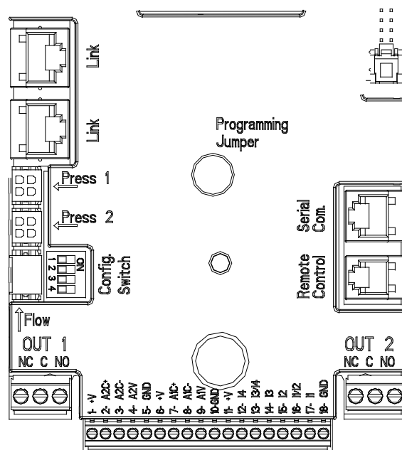
Figura 3: Conexiuni
