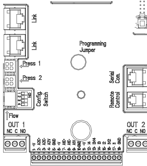
Resim 3: Bağlantılar
