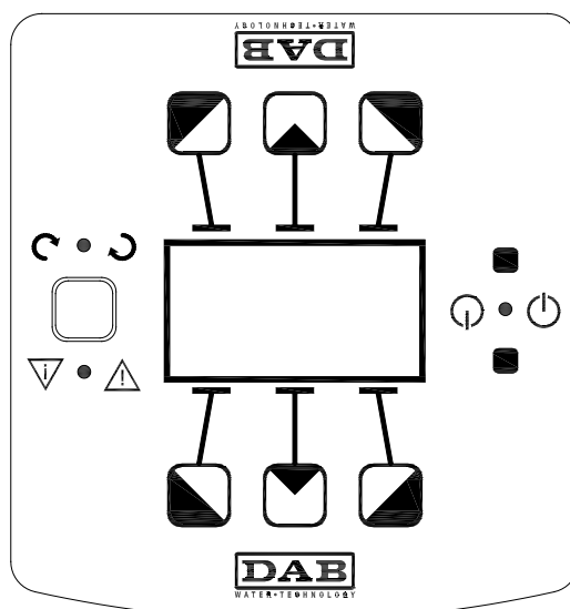
Fig. 10: Kontrollpanel
