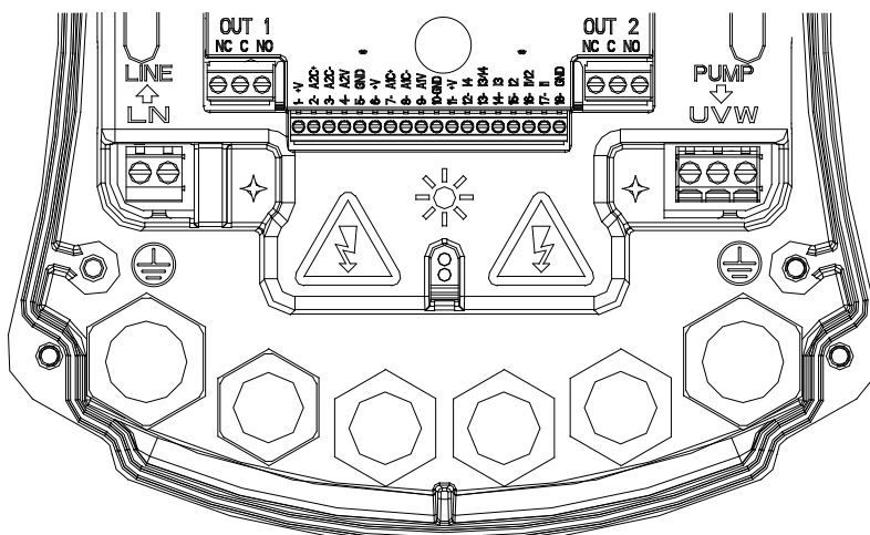
Figura 1: Conexiuni Electrice
