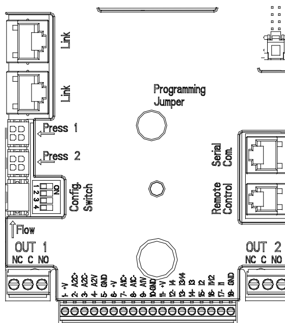
Abbildung 3: Anschlüsse
