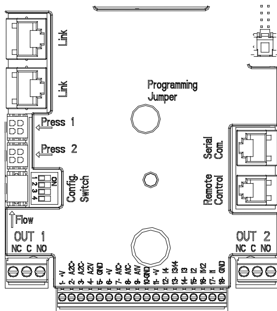
Схема 3: З'єднання
