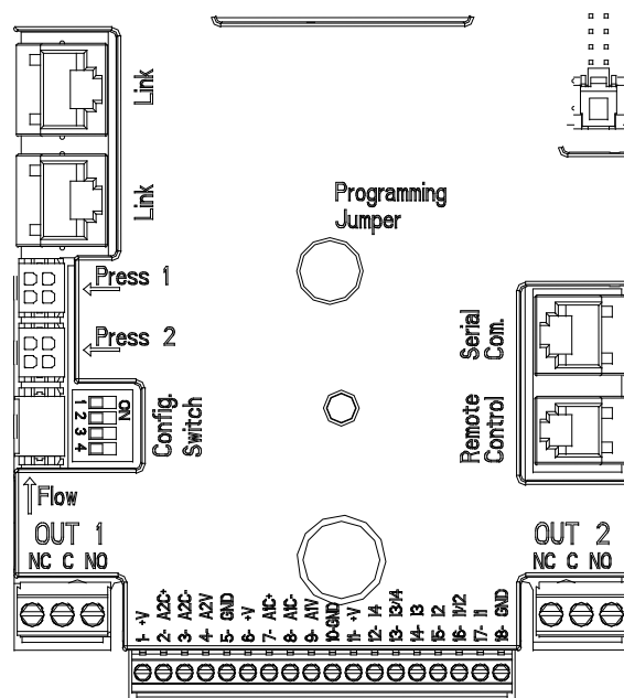
Figura 3: Conexiones
