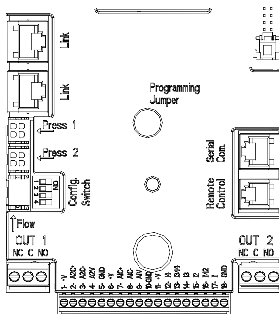
Afbeelding 3: Aansluitingen
