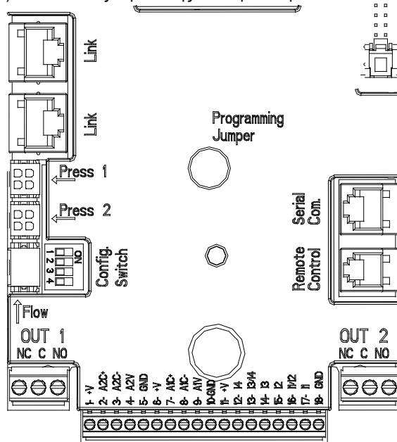
Σχήμα 3: Συνδέσεις
