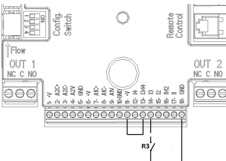
Figura 5: Esempio Collegamento Ingresso Digitale Quick Start
