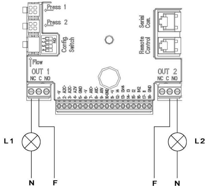
Abbildung 9: Anschlussbeispiel Digitalausgänge
