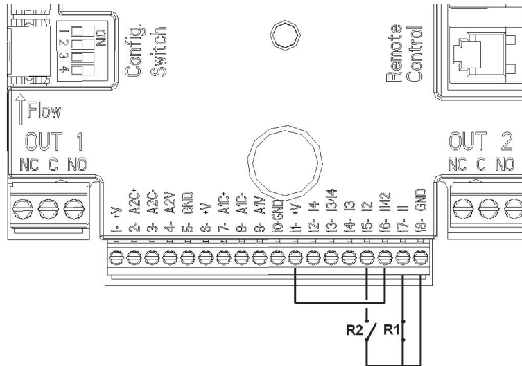
4 ábra: Start/Stop és Economy Digitális bemeneti bekötési példa
