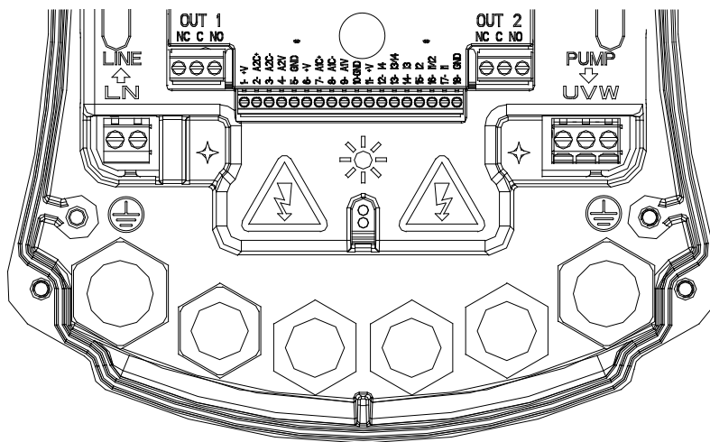
Slika 1: Električni priključki
