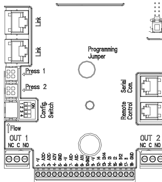
3.ábra: Csatlakozások
