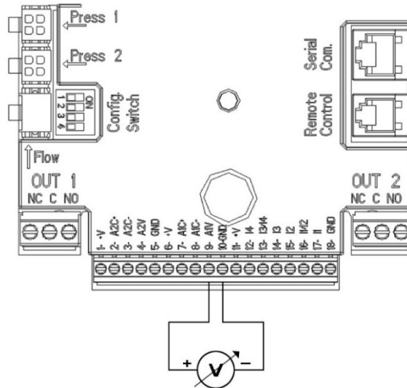
Figura 6: Exemplu Conexiune Intrare Analogica
