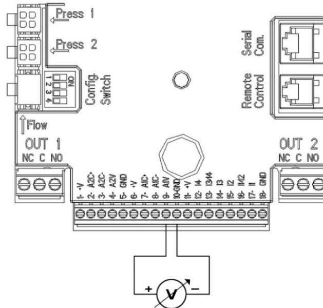
Figure 6: Exemple connexion entrée analogique
