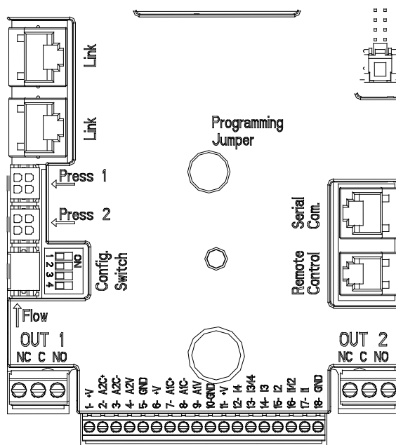
Схема 3: Соединения
