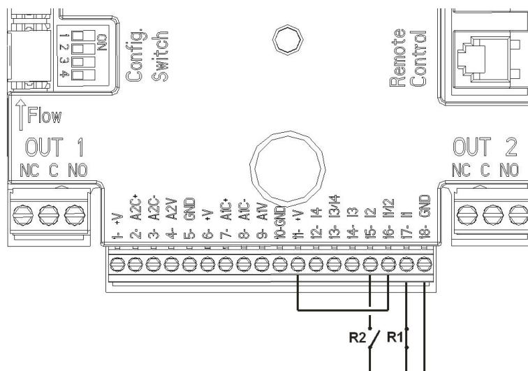
Fig. 4: Exempel på anslutning av digitala ingångar Start/Stop och Economy
